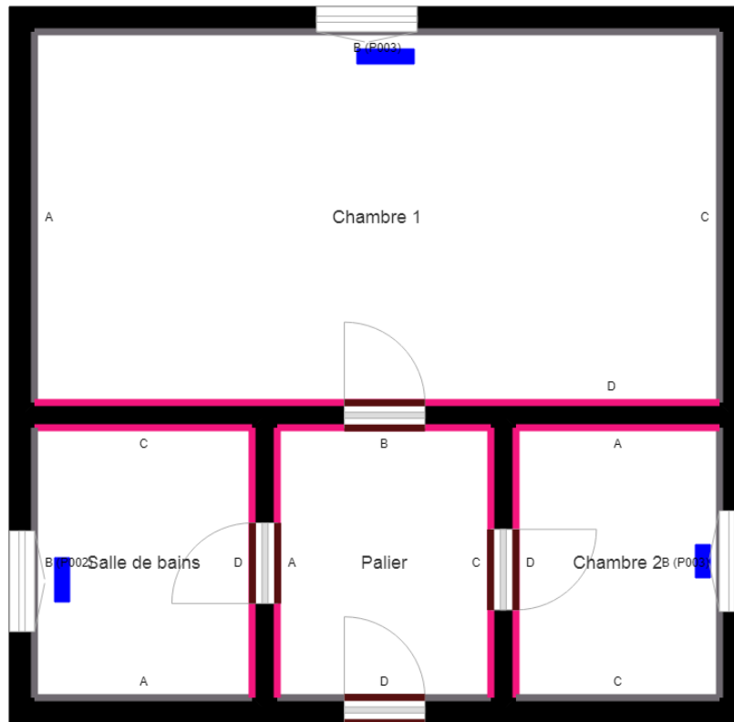
■ Convector électrique
